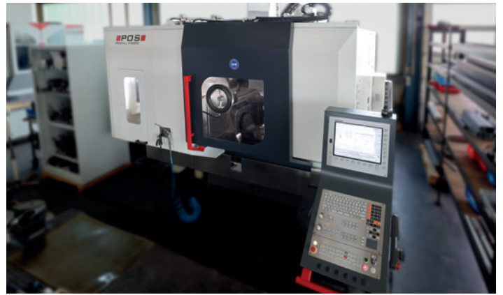
POS H500U X: 650 mm, Y: 750 mm, Z: 500 mm A: +/-120 °, C: 360 °, endlos, 5-Achs-Simultan Rundtisch Ø 500 mm, Heidenhain TNC 530
